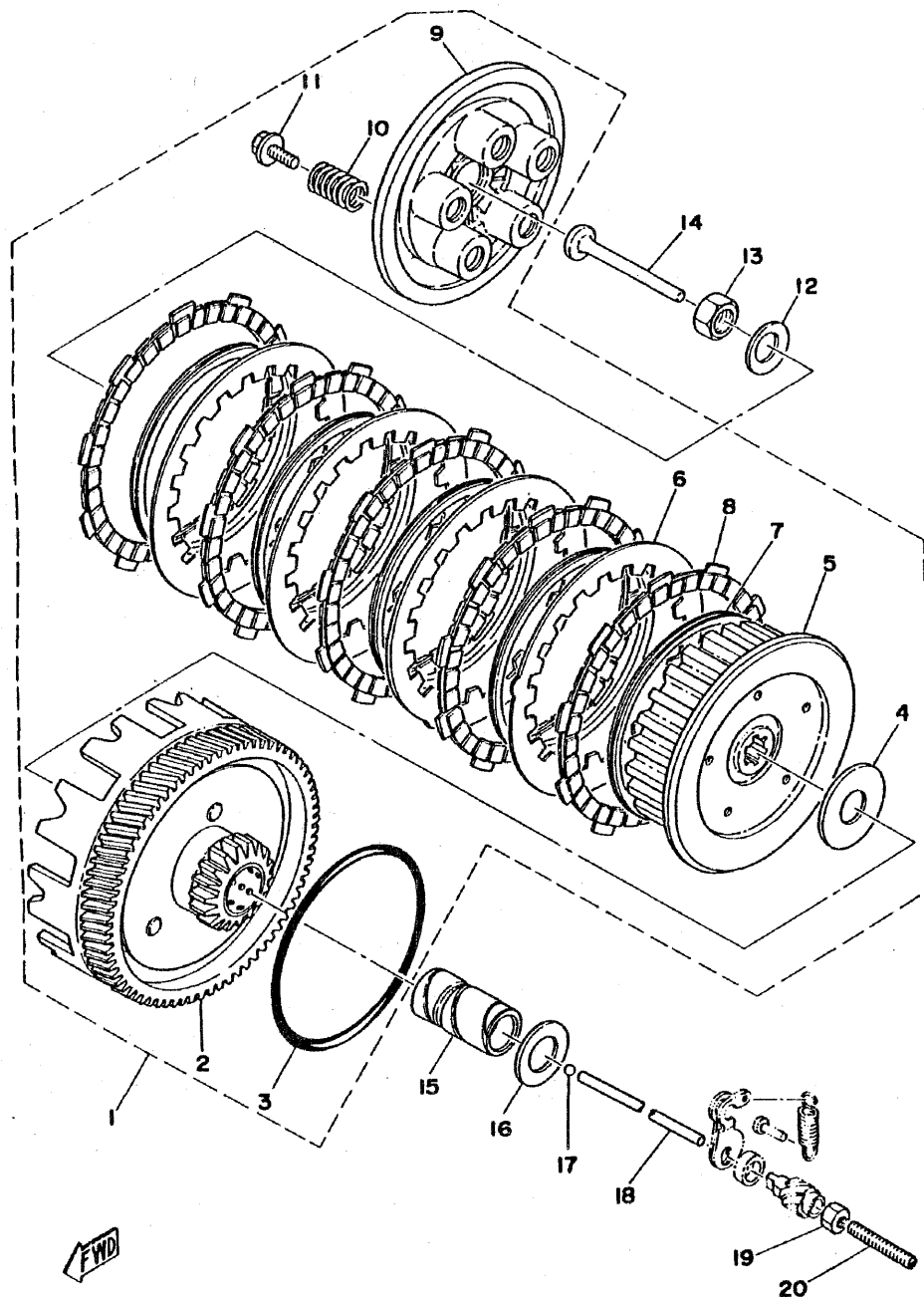
Fig. 4 CLUTCH
