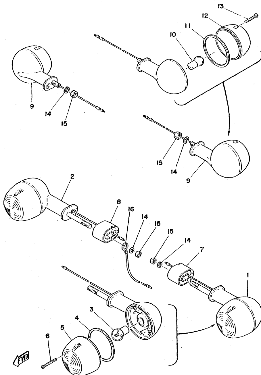
Fig. 35 FLASHER LAMP 1
