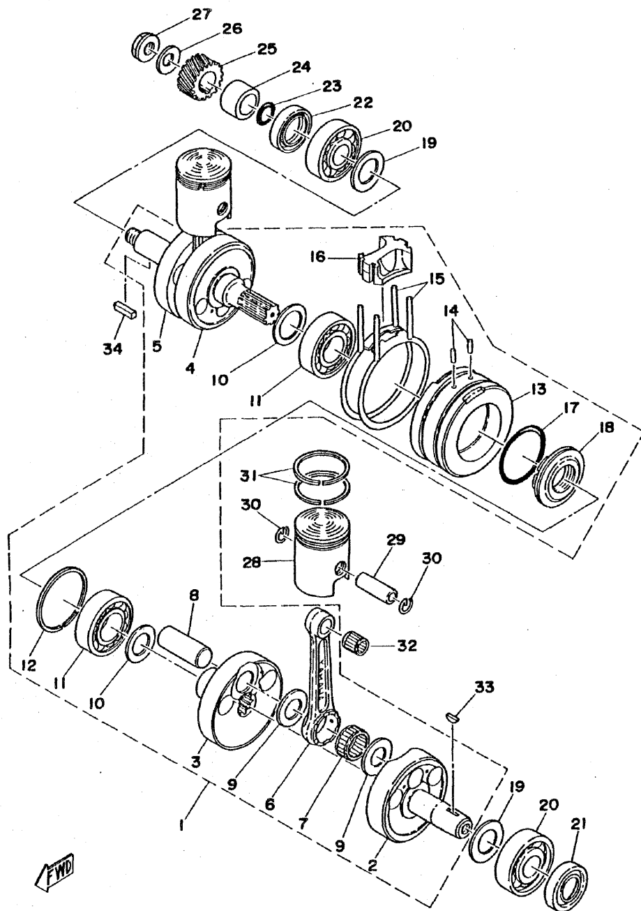
Fig. 3 CRANK · PISTON
