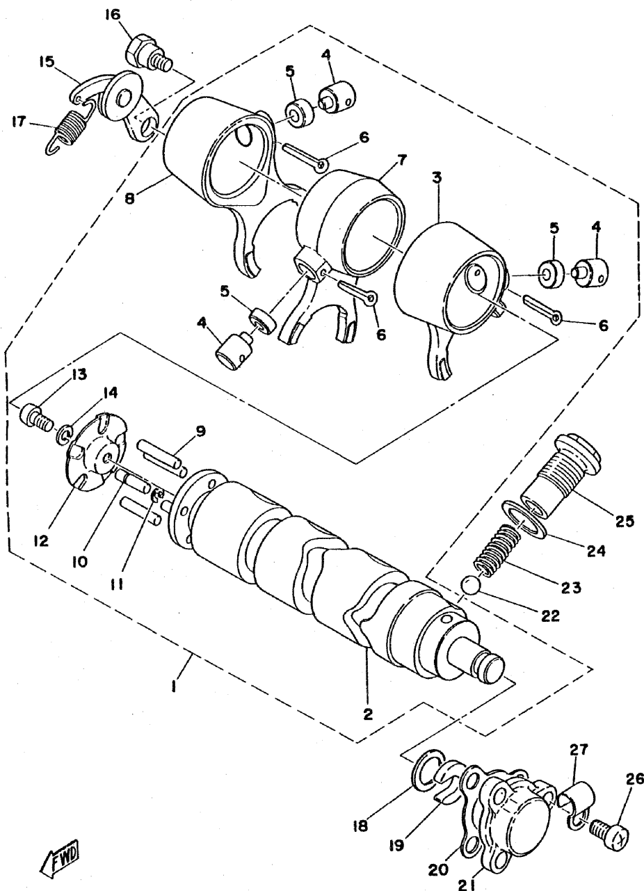
Fig. 6 SHIFTER 1
