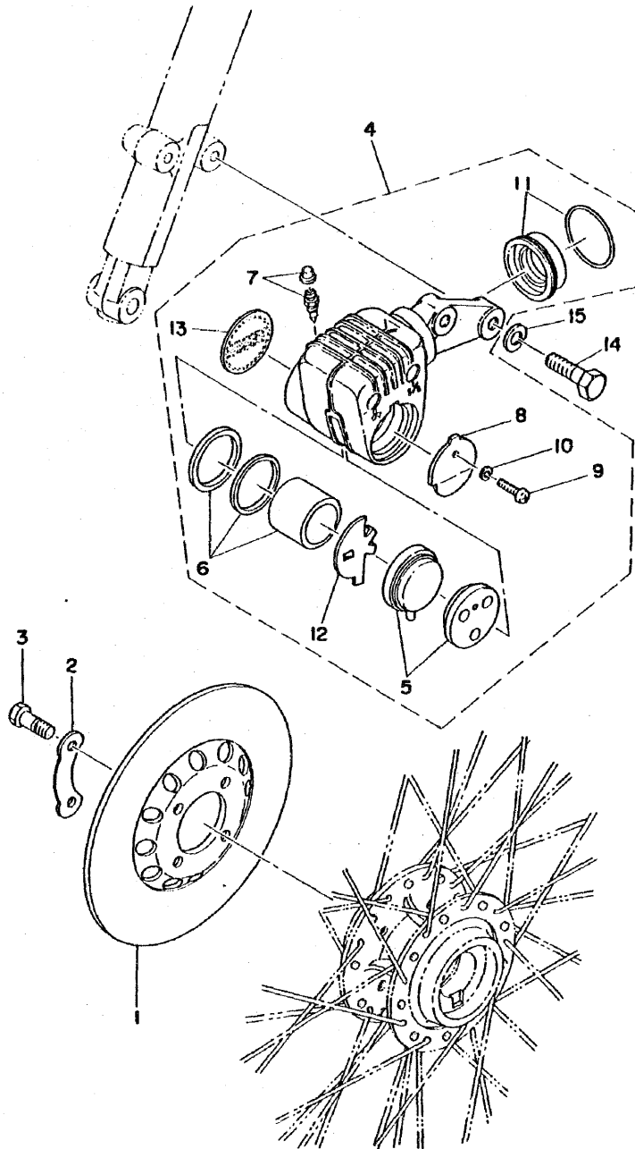
Fig. 28 DISK BRAKE · CALIPER
