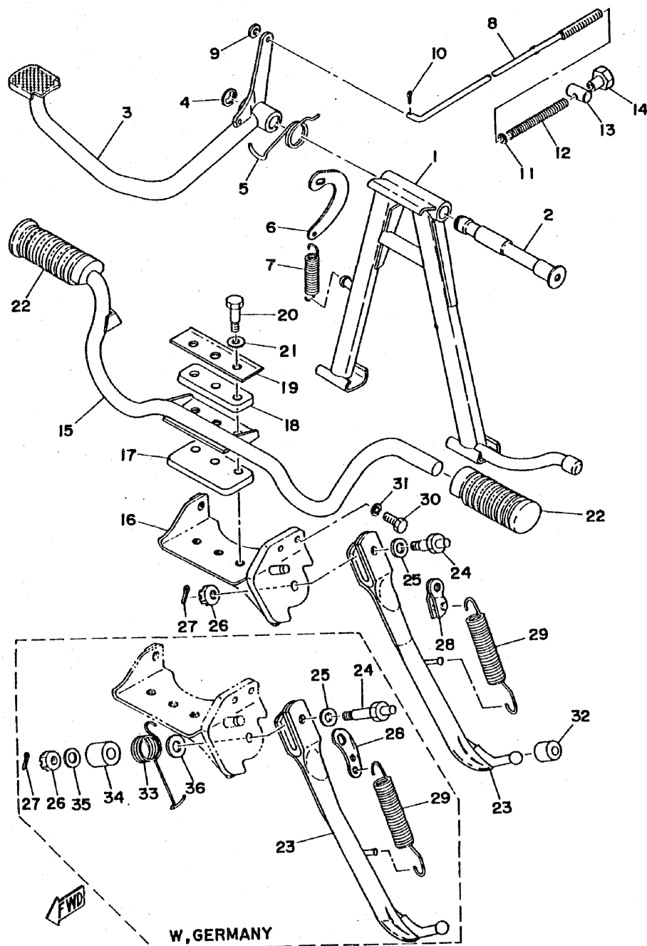
Fig. 18 STAND · FOOTREST · BRAKE PEDAL
