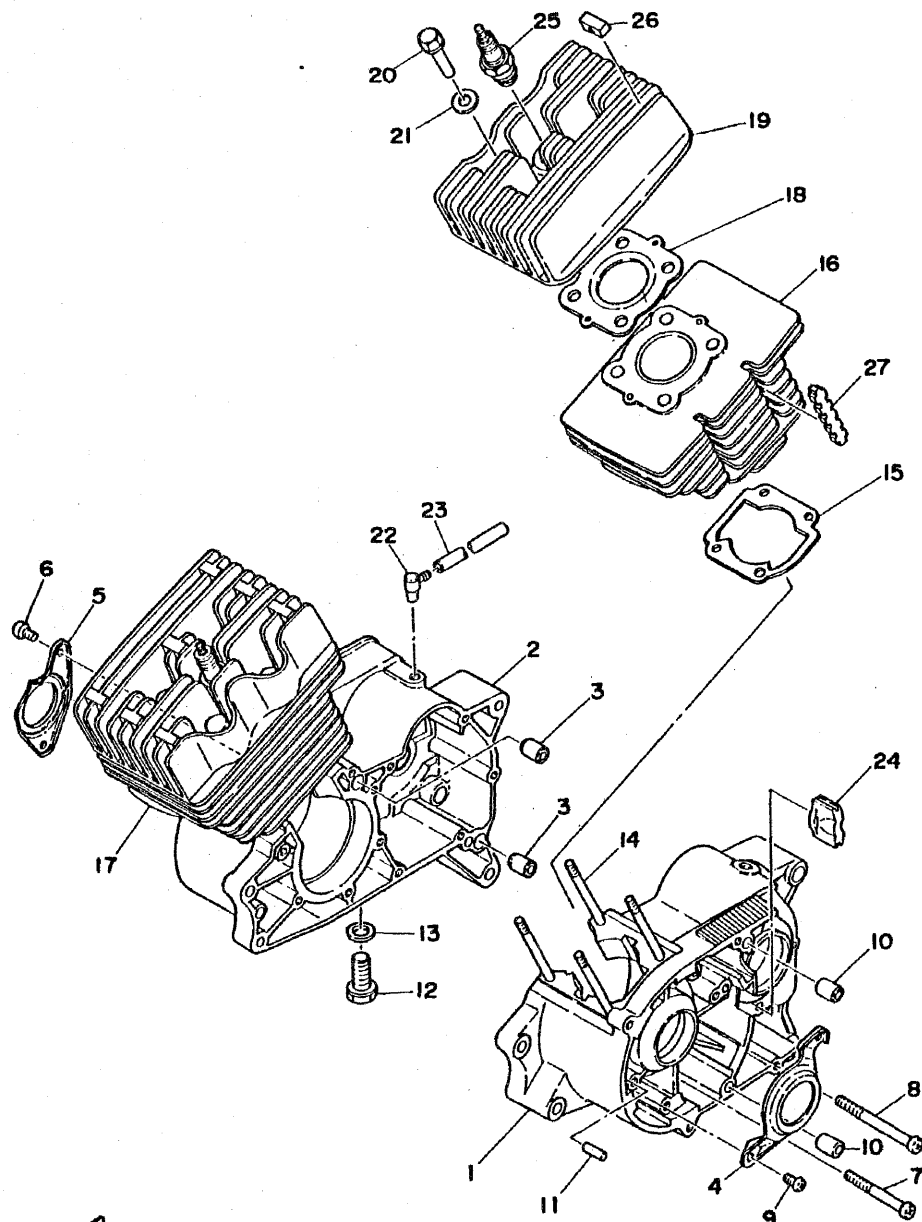
Fig. 1 CRANKCASE · CYLINDER
