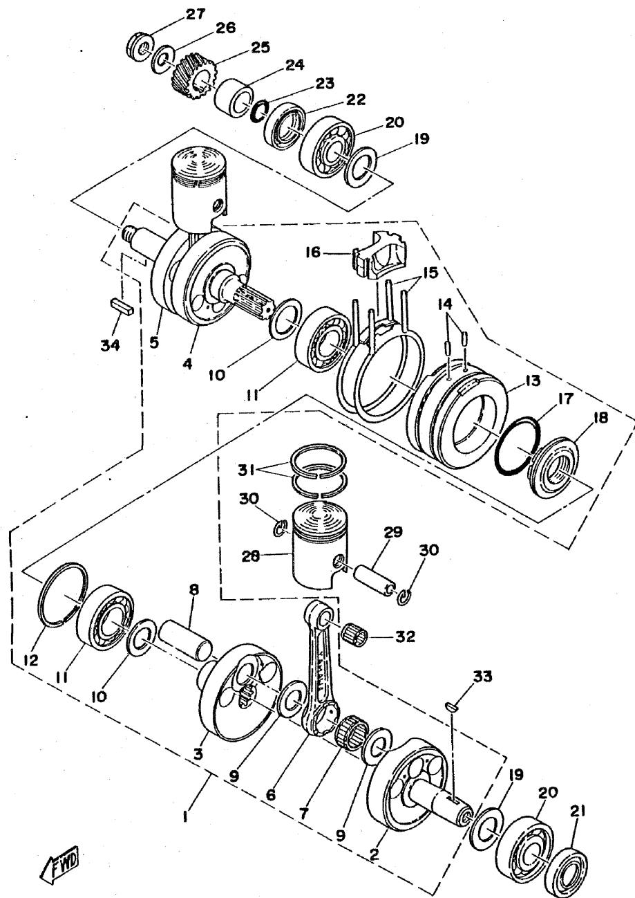
Fig. 3 CRANK · PISTON
